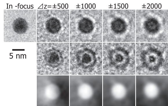
図1 金ナノ粒子のTEM像、および、位相像を示す。上段はアンダーフォーカス、中段はアンダーフォーカスのTEM像であり、下段は位相像である。左から右へデフォーカス値を500nmずつ増やした結果である 25) 。
